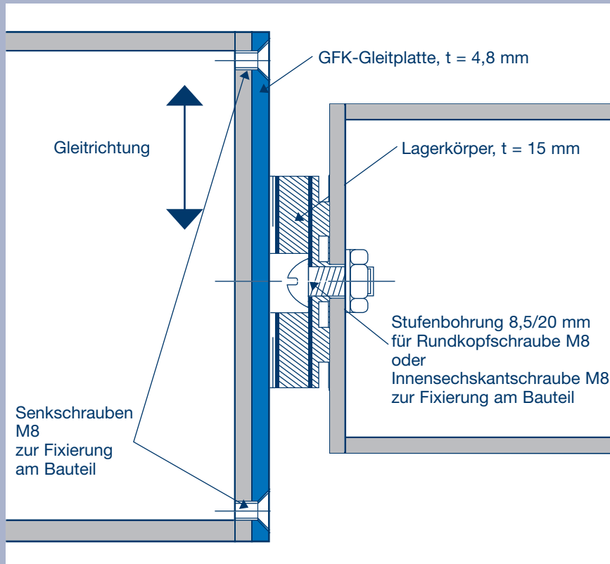
Bild 5: Einbaubeispiel eines Ciparal®-Gleitlagers ST, t = 20 mm, Vertikalfuge zwischen zwei Stahlbauteilen mit Befestigung der einzelnen Lagerkomponenten an den angrenzenden Bauteilen
